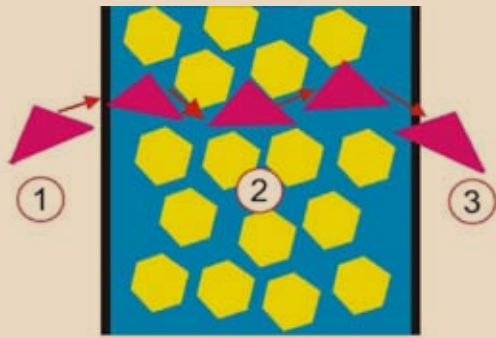
1 - Сорбция молекул пенетранта на наружной поверхности стенки полимерной трубы 2 - Диффузия сорбированных молекул пенетранта через стенку полимерной трубы 3 - Дисорбция молекул пенетранта в питьевую воду от противоположной (внутренней) поверхности стенки полимерной трубы
