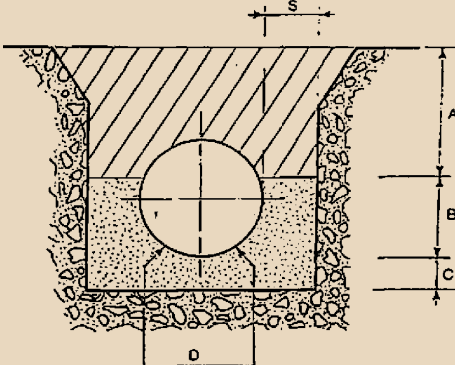
Рисунок 3. А – природный материал засыпки; В – подложка, минимум 70% от диаметра трубы; С – подушка, минимум 15 см; D – устойчивая опора должна обеспечиваться в этих точках; S – 60 см. минимум
