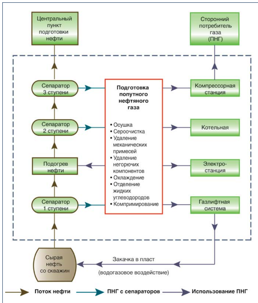
Рис. 1. Рациональное использование попутного газа
