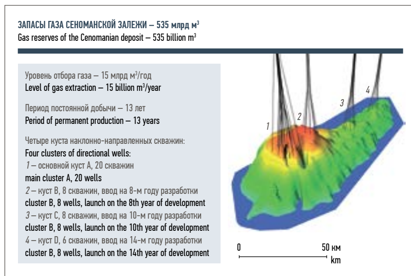
Рис. 3. Перспективы ввода объектов месторождения Каменномысское-море Fig. 3. Prospects for starting facilities of the Kamennomysskoye-mоре field
