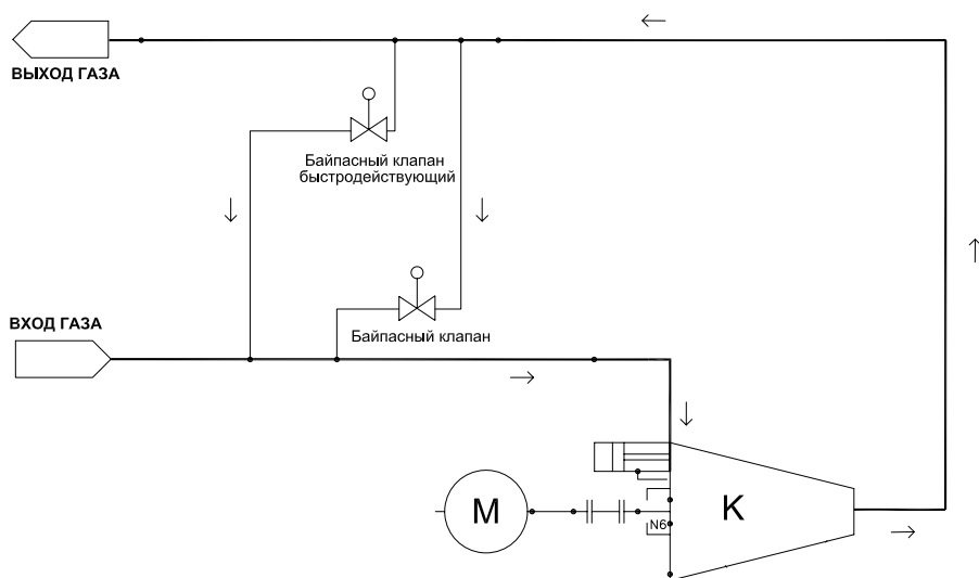
Рис. 1. Принципиальная схема байпасной линии
