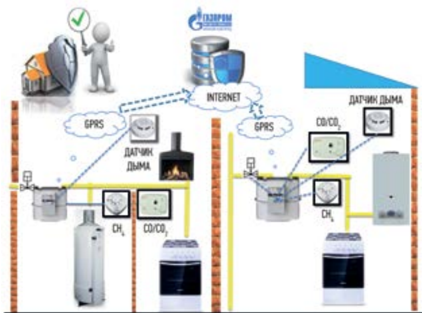
Рис. 2. Схема обеспечения безопасности эксплуатации ВДГО и ВКГО
